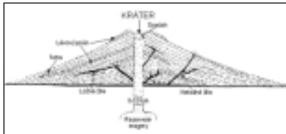
Obr. 2: Stratovulkánická stavba sopečných aparátov Slanských vrchov.
