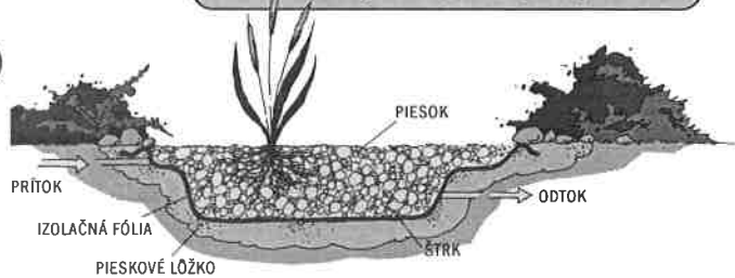
Obr. 4: Biologická čistička odpadových vôd
