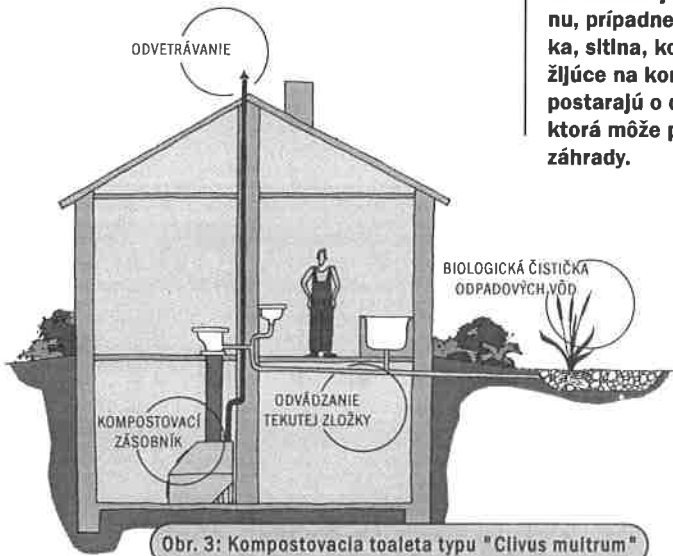
Obr. 3: Kompostovacia toaleta typu "Clivus multitrans"
